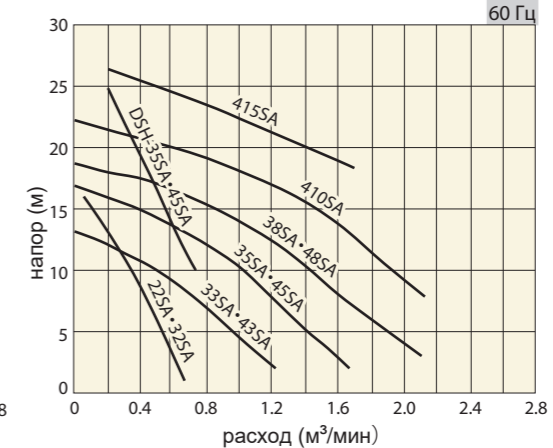
DS-415SA (фланцевое соединение)
