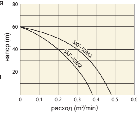
◆ диаграмма производительности
